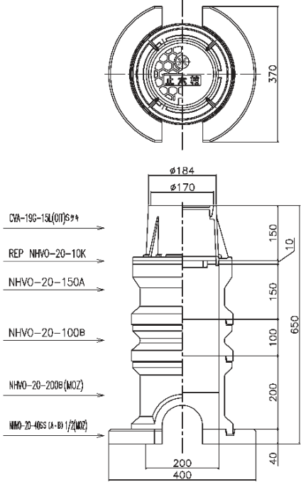
仕切弁室標準図 S=Free(切欠付)
