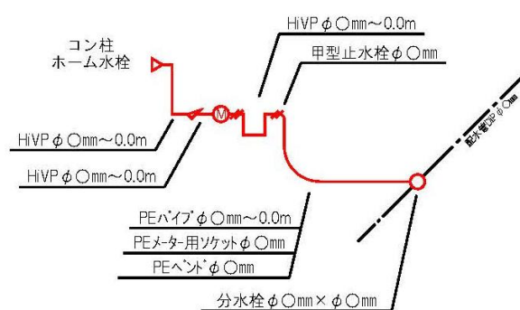
立面図
