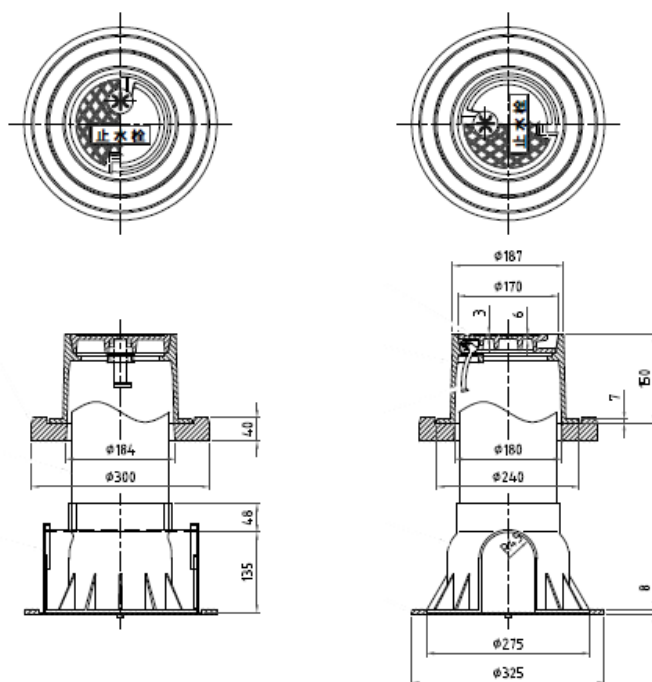
止水栓ボックス 2号(大)―車道等
