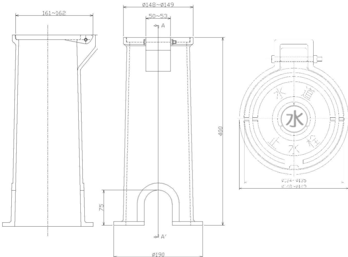
<止水栓ボックス T-8 標準図>
