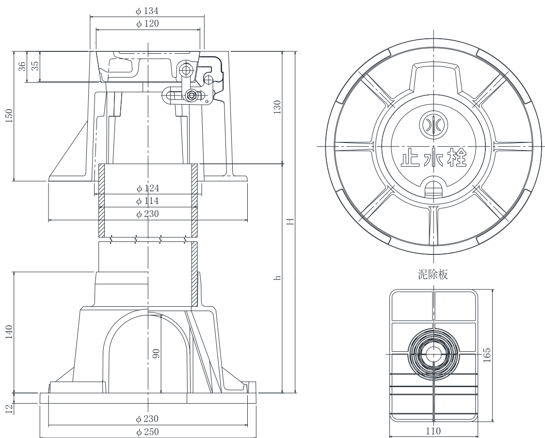
＜止水栓ボックス T-14(C 形 2 号) 標準図＞
