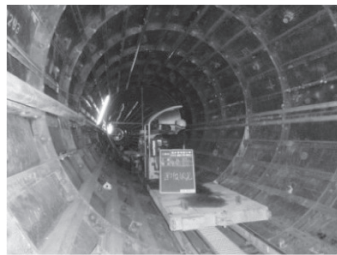
バイパス送水管の整備 など主要管路の2重化
