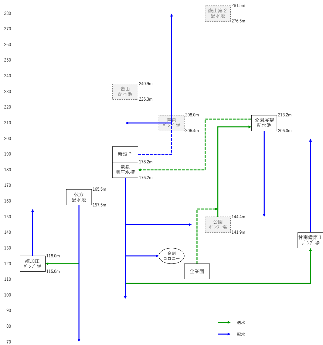
図 3.20 対象地域の送配水フロー（計画：第1段階）
