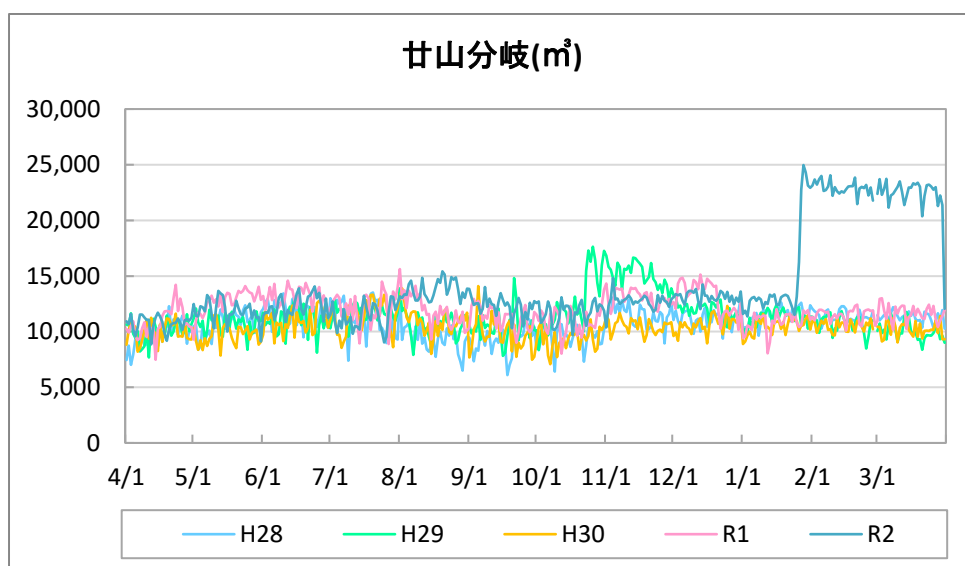
図 3.5 甘山分岐受水量（平成 28～令和 2 年度）
