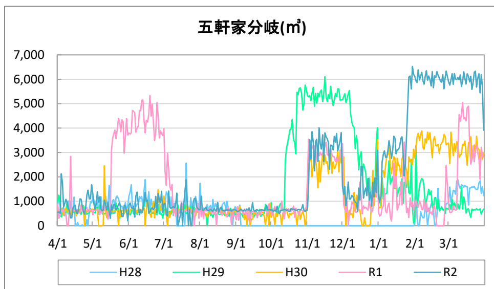
図 3.6 五軒家分岐受水量（平成 28～令和 2 年度）
