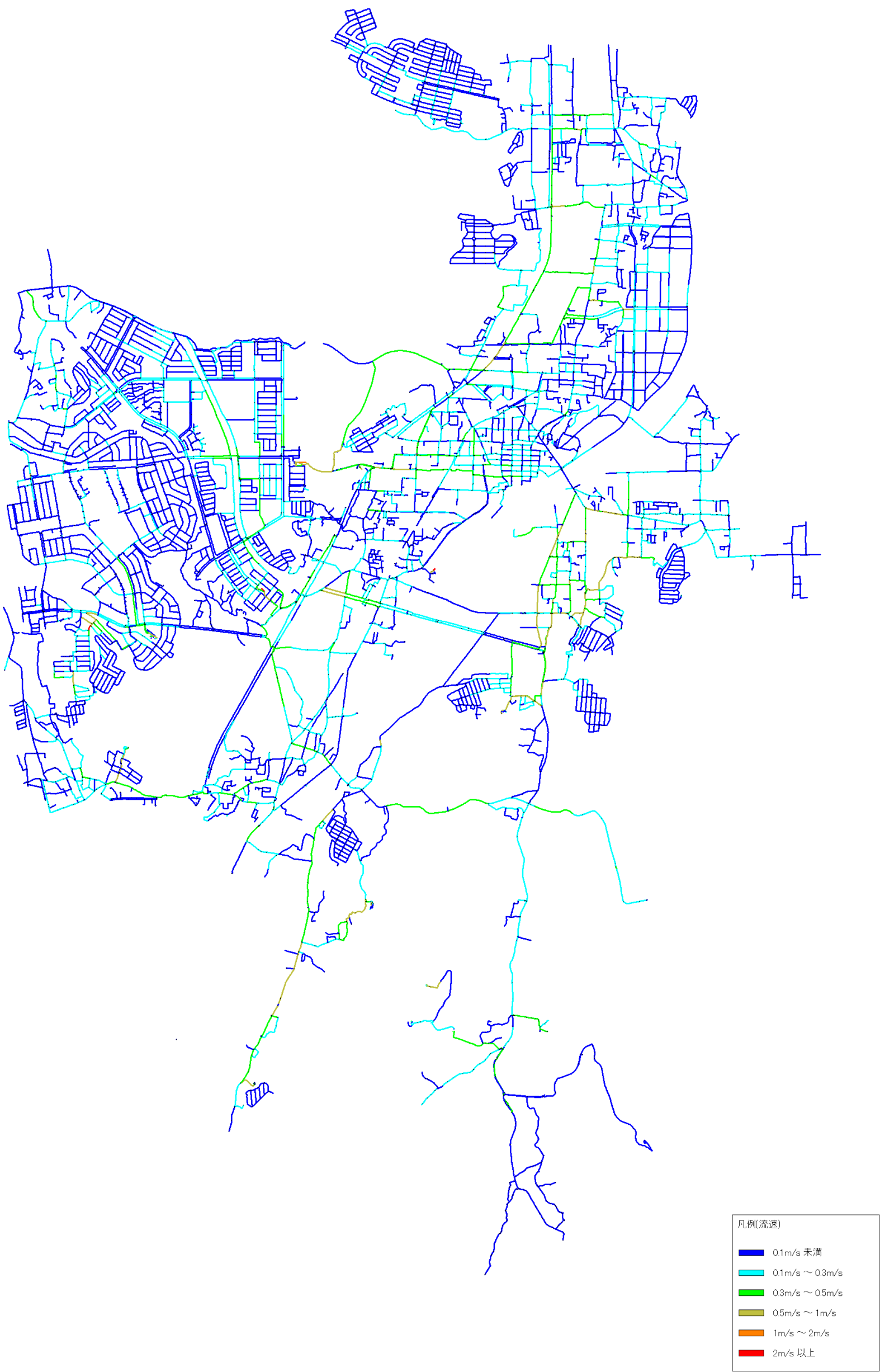
図 3.12 配水管の流速
