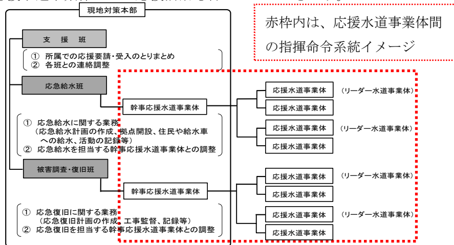
図-3 指揮命令系統イメージ図
