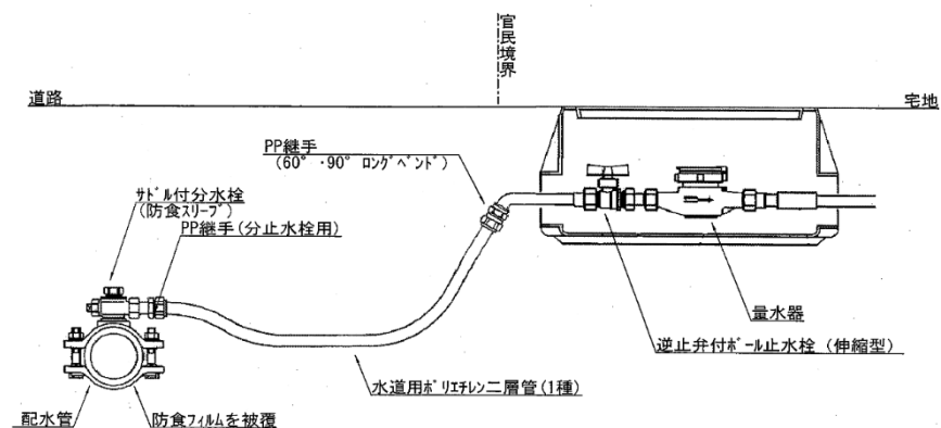
図-10 給水管の標準構造図
