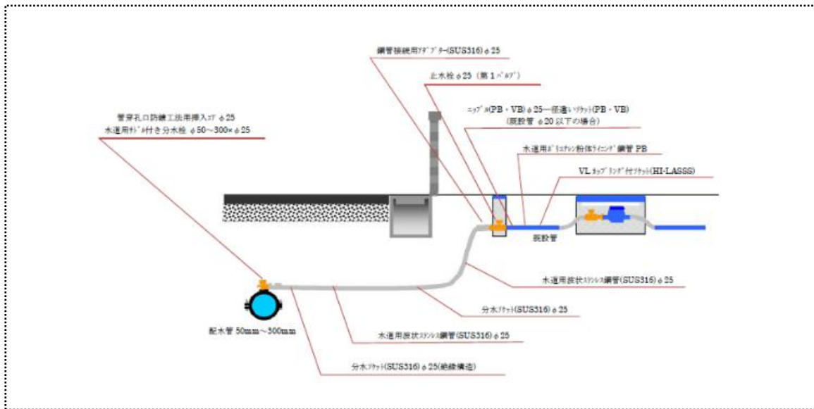
図-10 給水管の標準構造図
