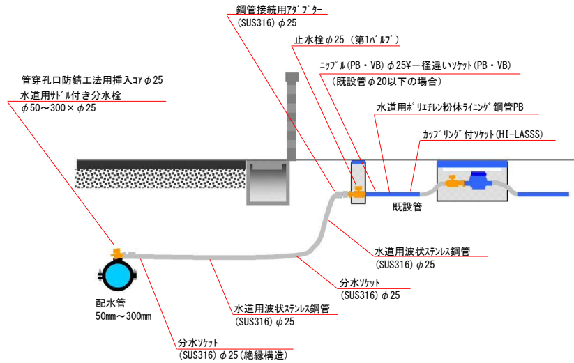
図-10 給水管の標準構造図
