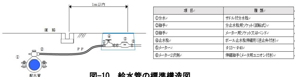
図-10 給水管の標準構造図
