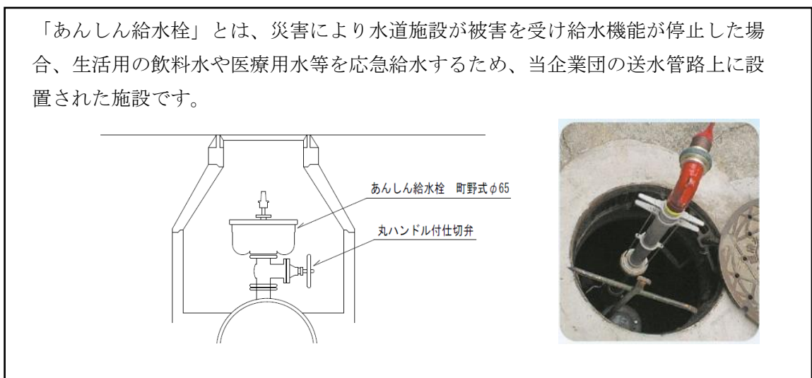
図-5 あんしん給水栓について
