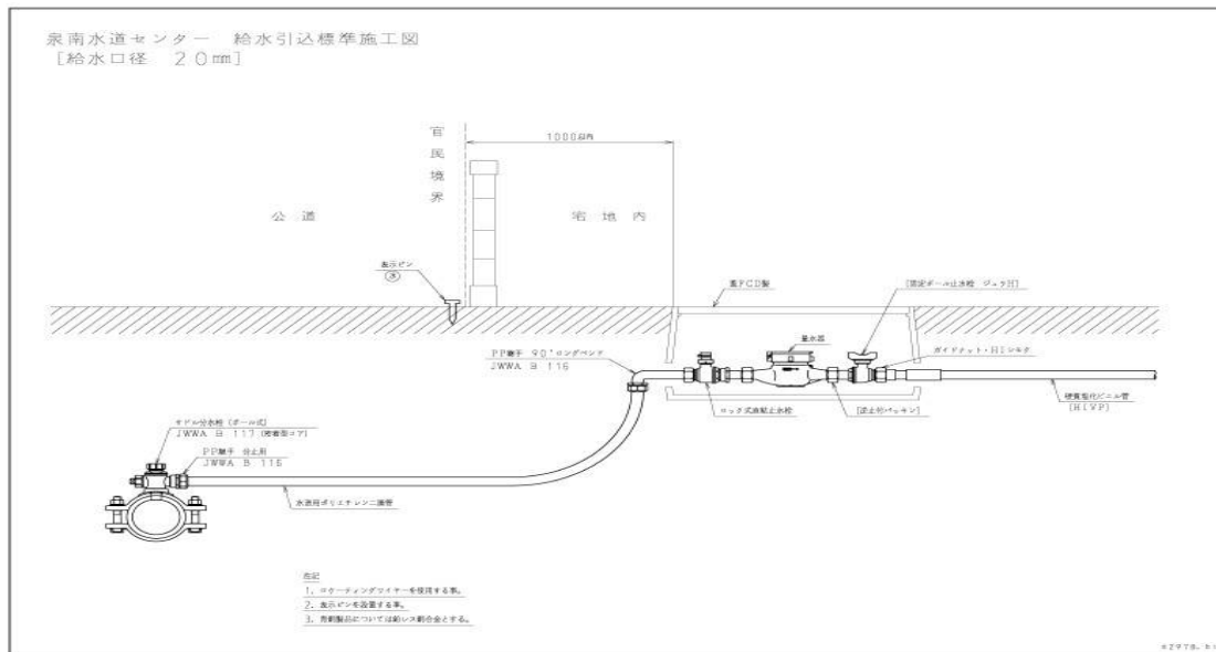
図-10 給水管の標準構造図
