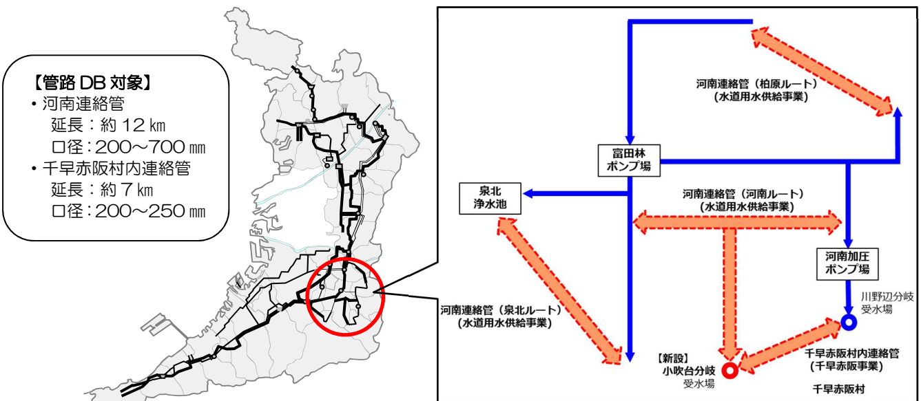
河南連絡管・千早赤阪村内連絡管 対象箇所図
