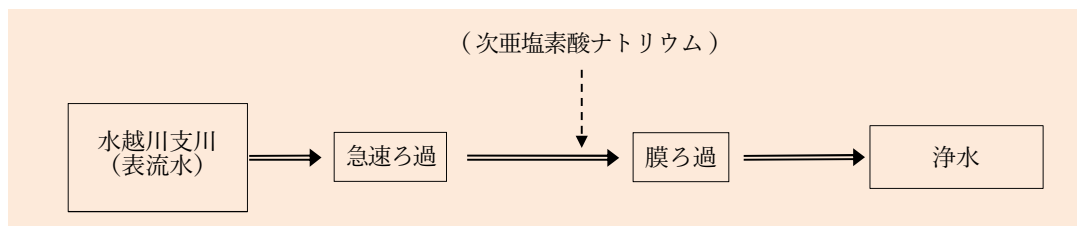
図 浄水場の処理フロー
