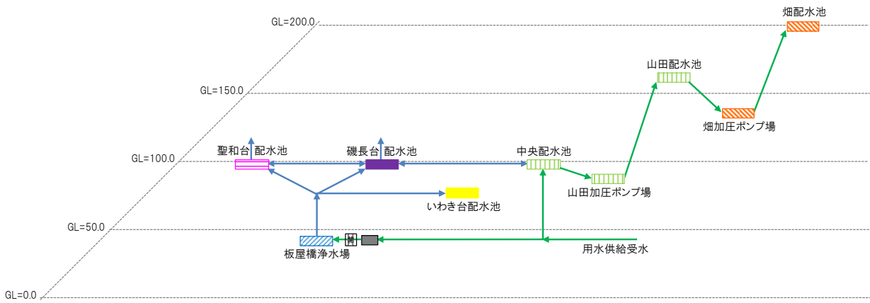
図2 送配水系統図
