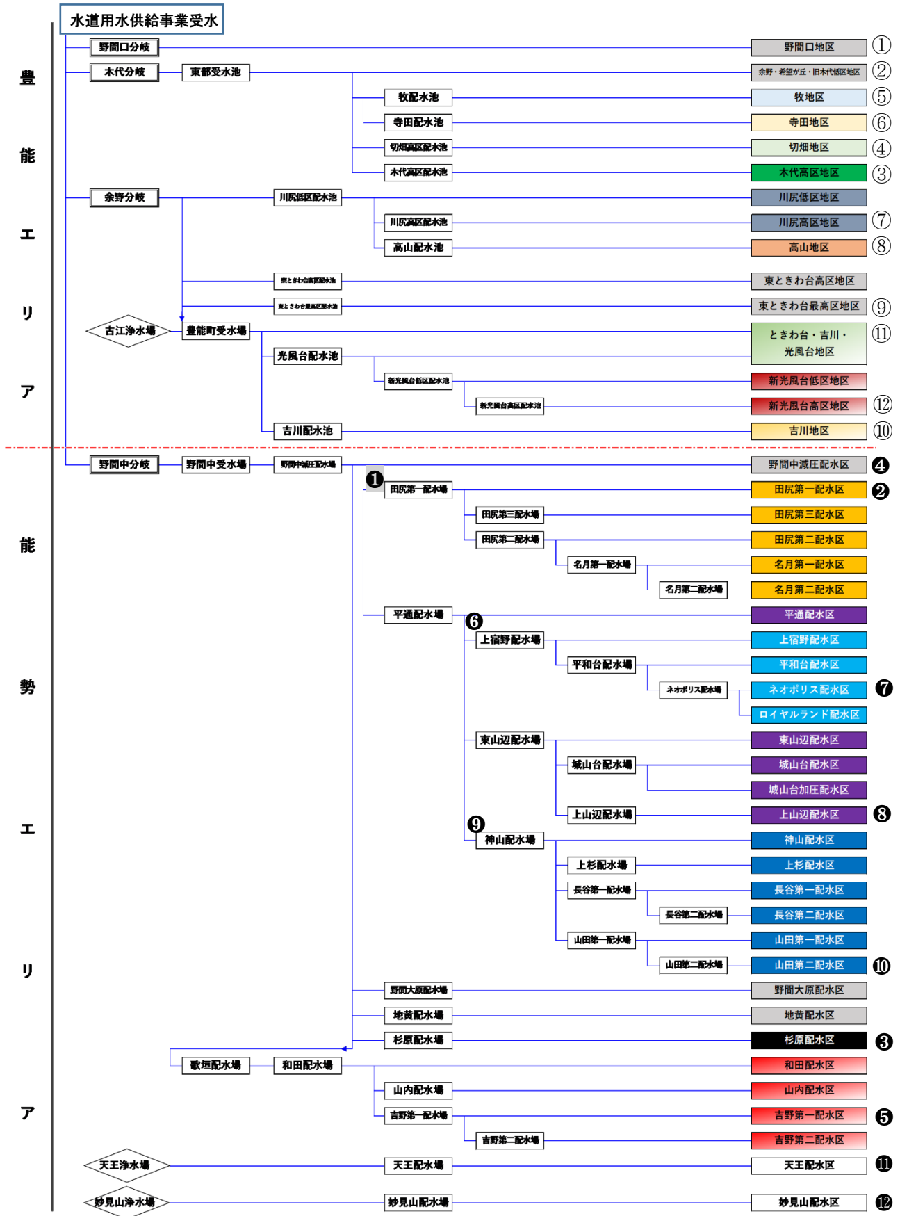
図 1 配水系統図
