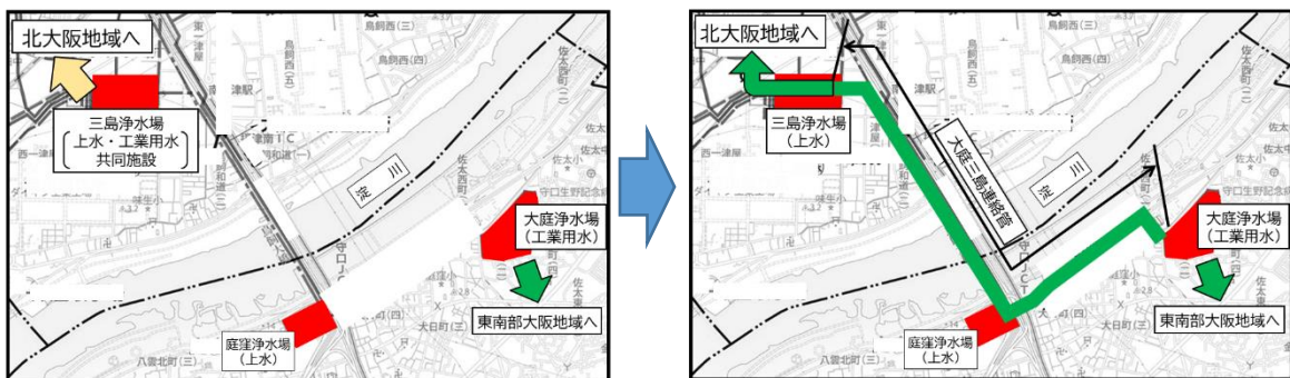
大庭浄水場一元化後の配水形態
