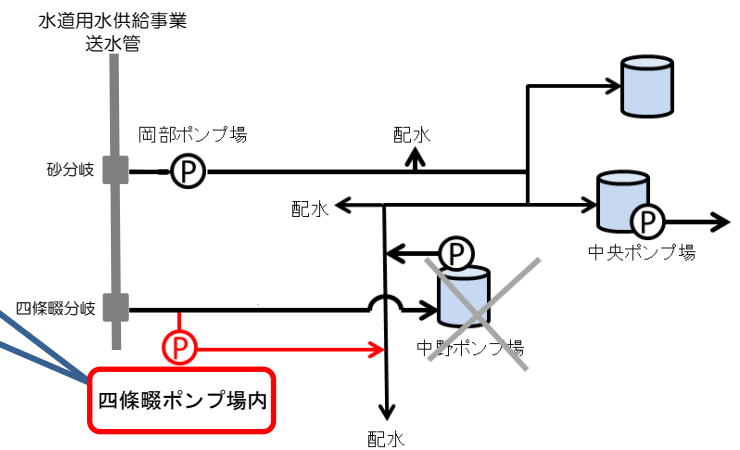
四條畷水道事業の送配水計画の系統図
