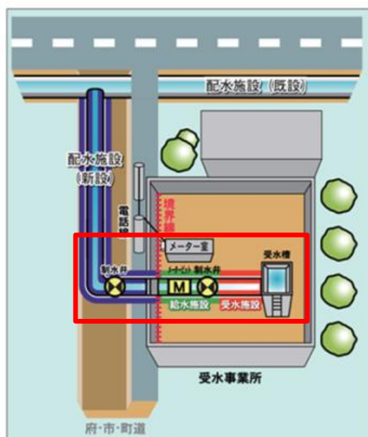
工業用水道メーター設置概要図
