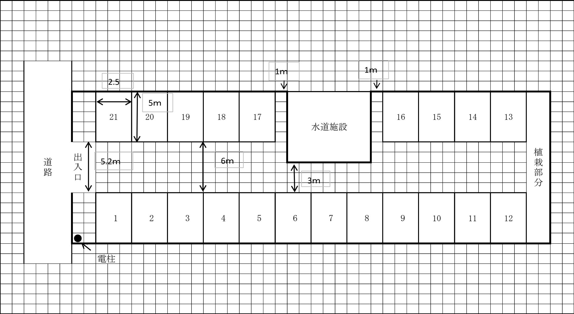
計画概要図
