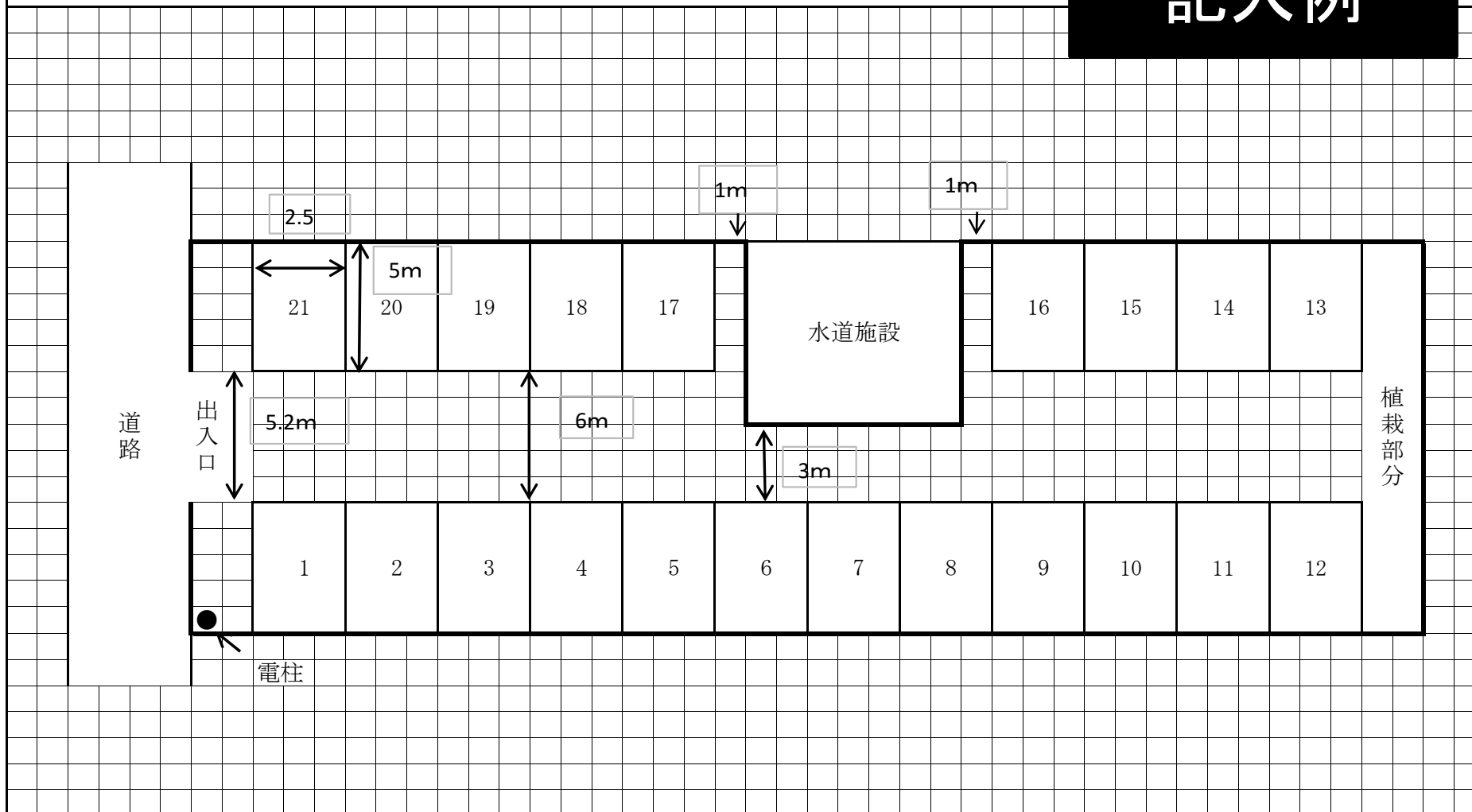
計画概要図
