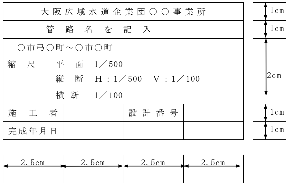
図1-3 表題欄の寸法及び様式
