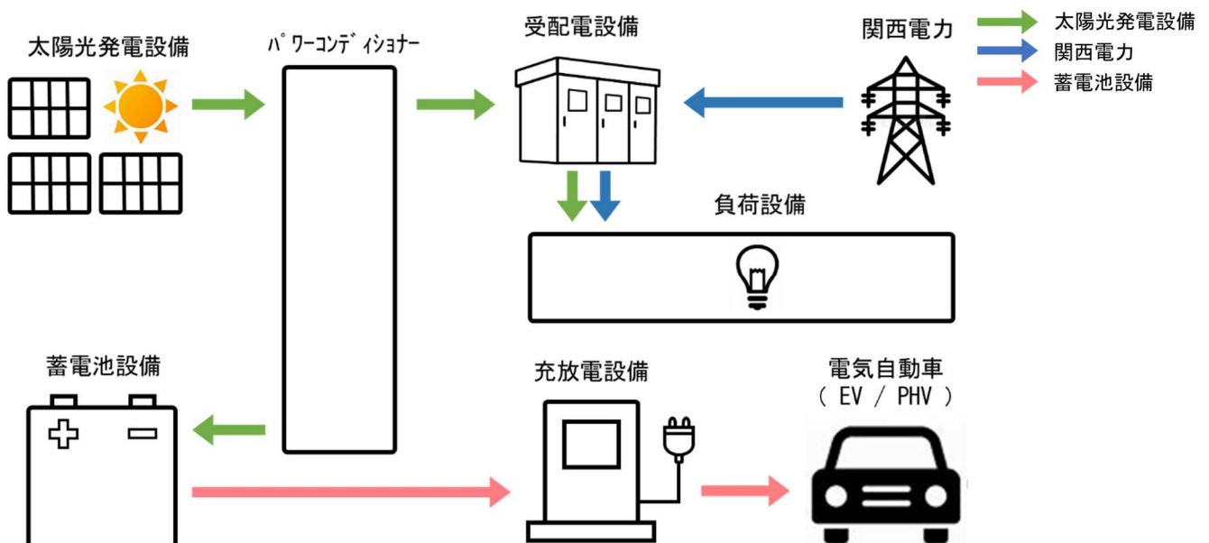
太陽光発電設備のシステム概要（通常時）
