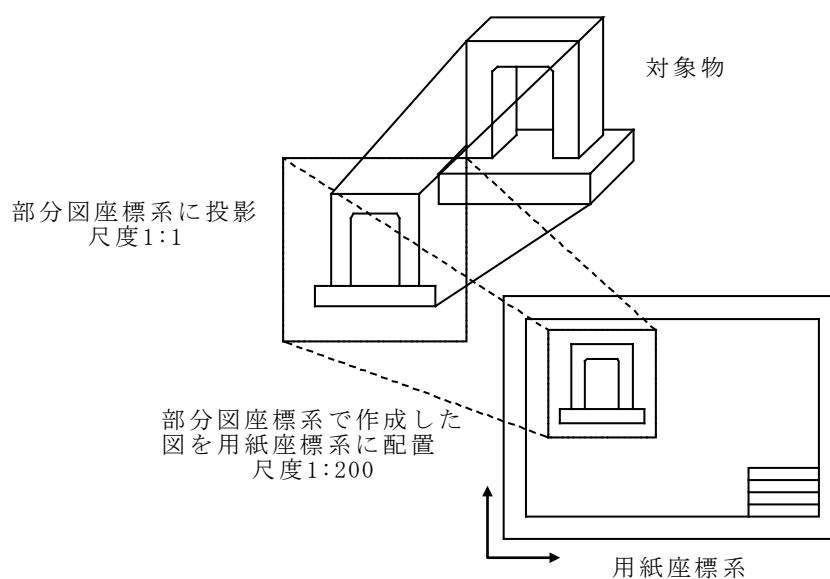
解説 図1-18 用紙座標系と部分座標系の関係
