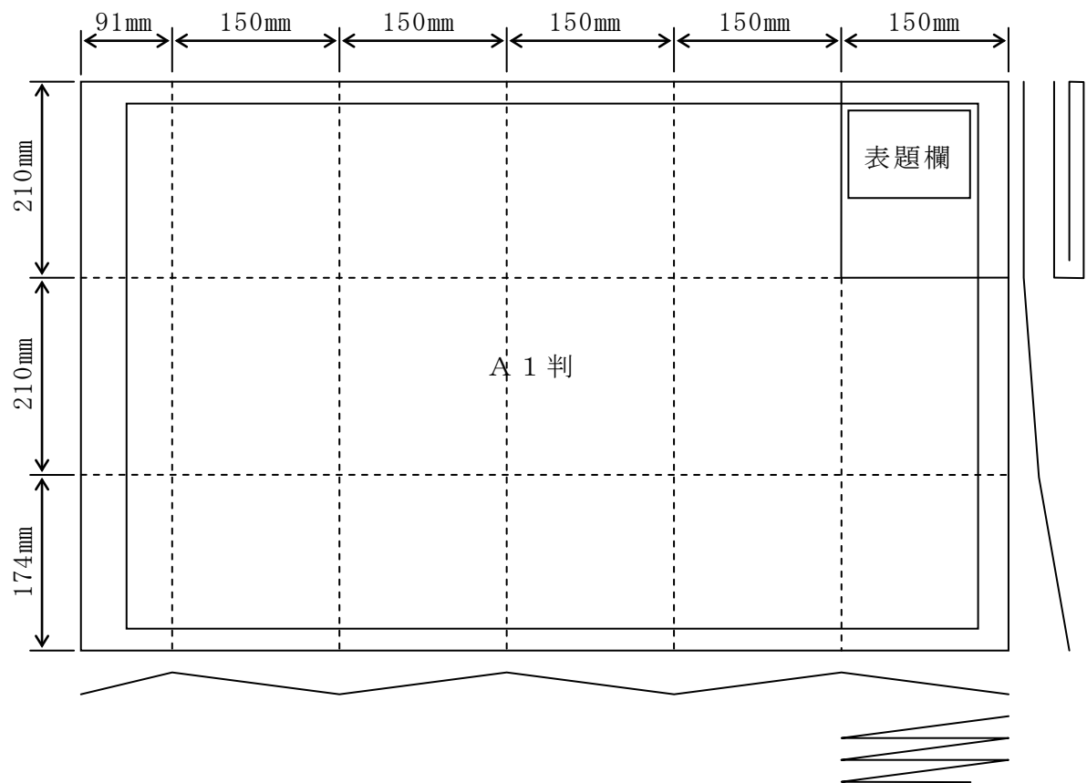
図1-4 図面の構成
