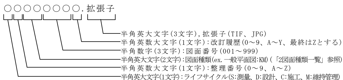
図1-14 ラスタファイルの命名規則(SXF Ver. 3.0レベル2の場合)
