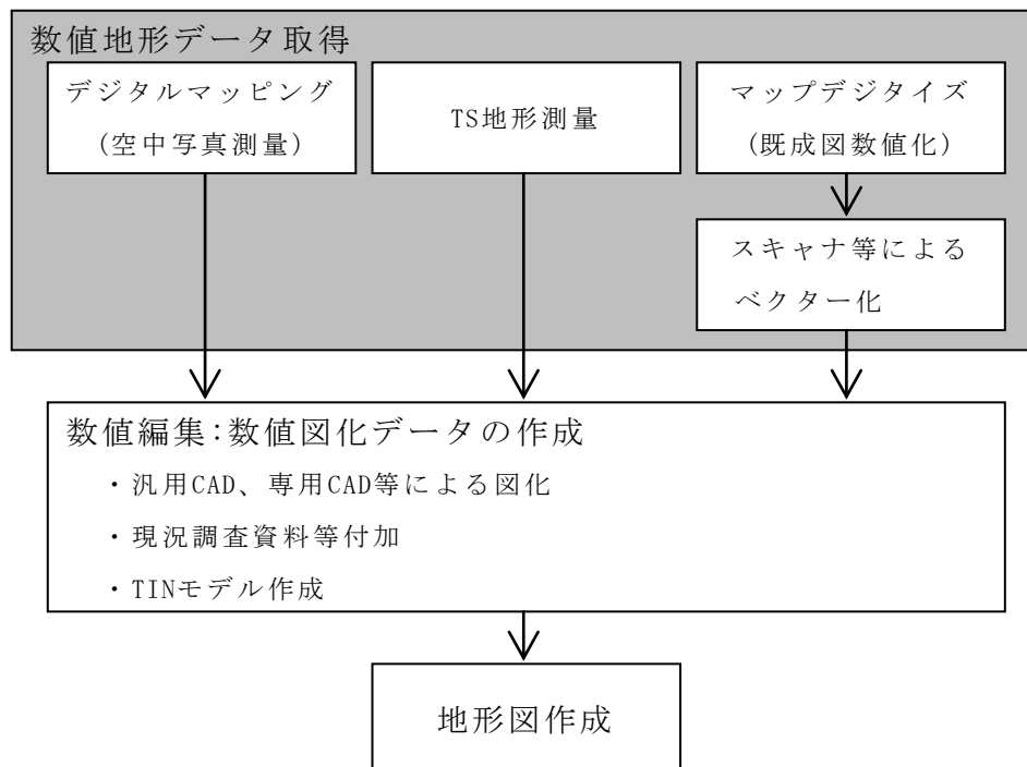
図3-1 地形図作成までのプロセス
