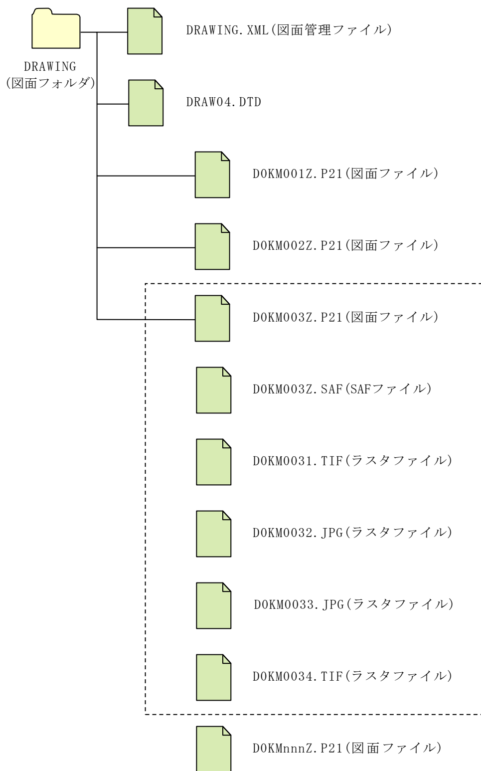
解説 図1-16 SXF Ver. 3.0 レベル2以上でのラスタファイルの格納例 (設計業務等の場合)
