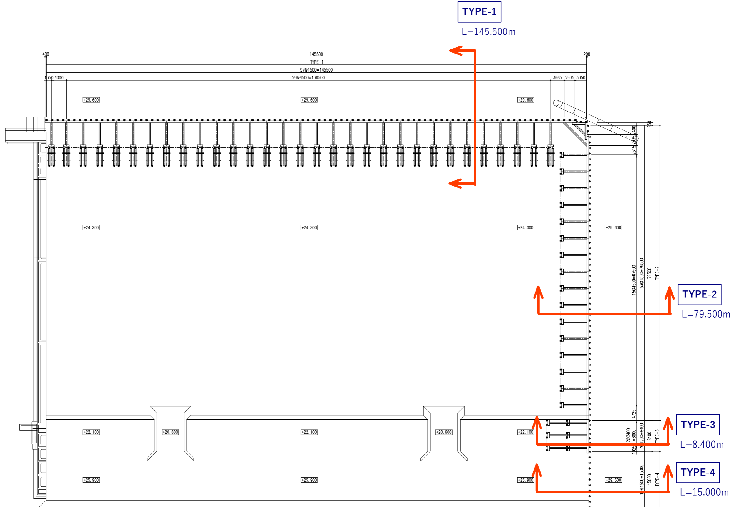
平面図
